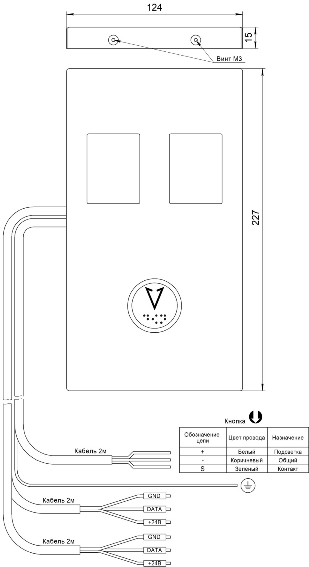
Рис.1 Внешний вид, габаритные и установочные размеры Вызывного поста КВАДРО НШЕК.468381.068-01
